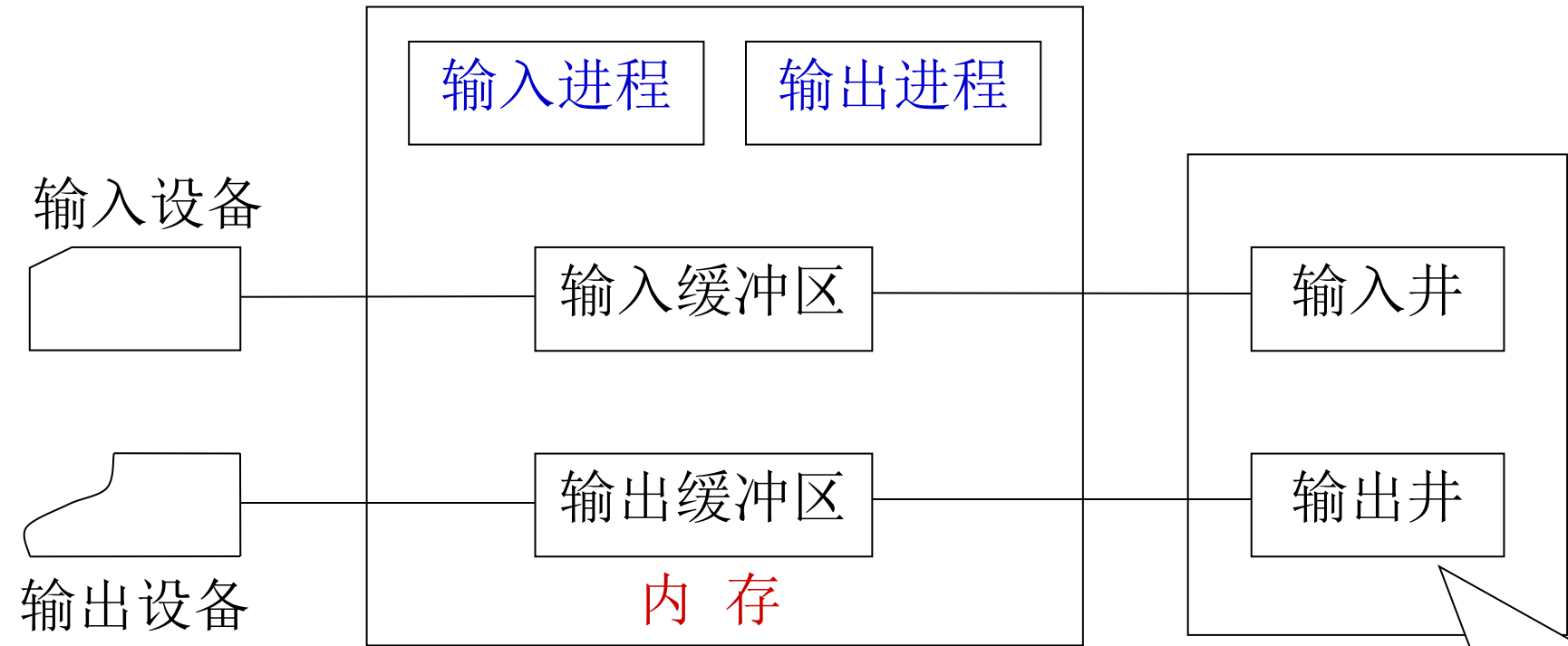
SPOOLING系统的组成
